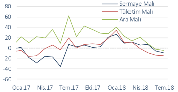
Geniş Ekonomik Sınıflandırmaya Göre İthalat (yıllık % değişim)
